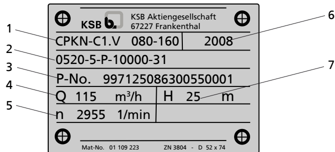
Рисунок 4: Заводская табличка
