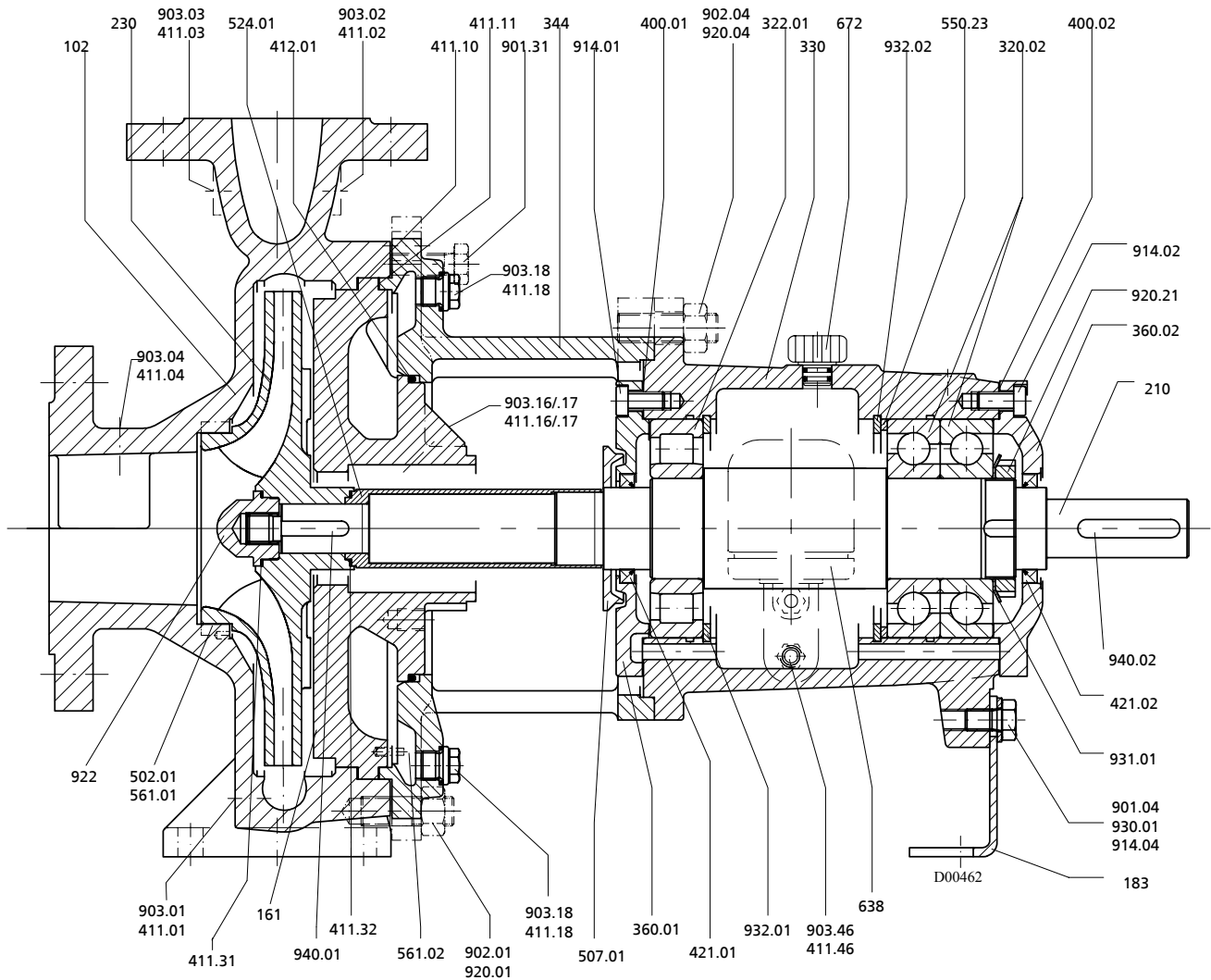
Рисунок 17: Общий чертеж стандартного исполнения (с масляной смазкой)
