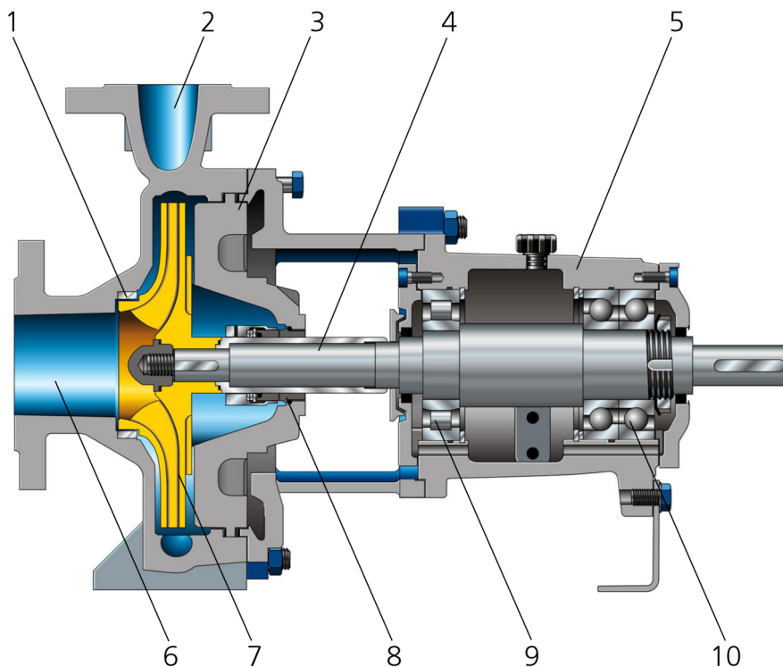
Рисунок 5: в разрезе
