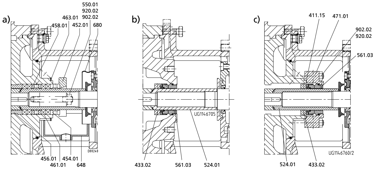
Рисунок 18: Исполнение с сальниковой набивкой (а), торцевое уплотнение с конической крышкой корпуса (b), торцевое уплотнение с цилиндрической крышкой корпуса (с)
