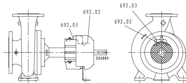
Рисунок 4: Подключения НРК-L
