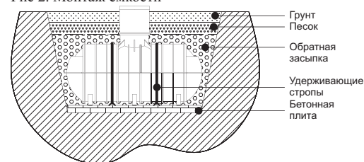
Рис 2. Монтаж емкости
