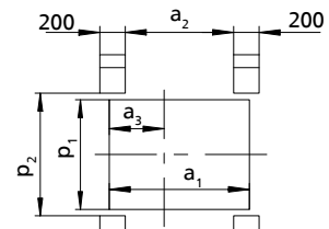
Foundation holes 71)
