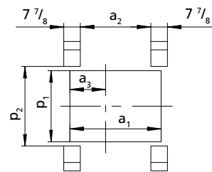
Foundation holes 28)
